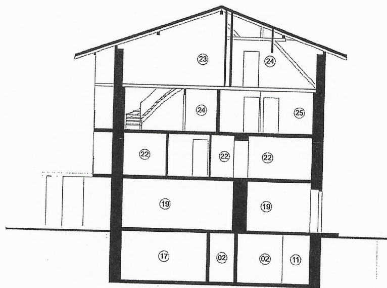
Coupe AA
